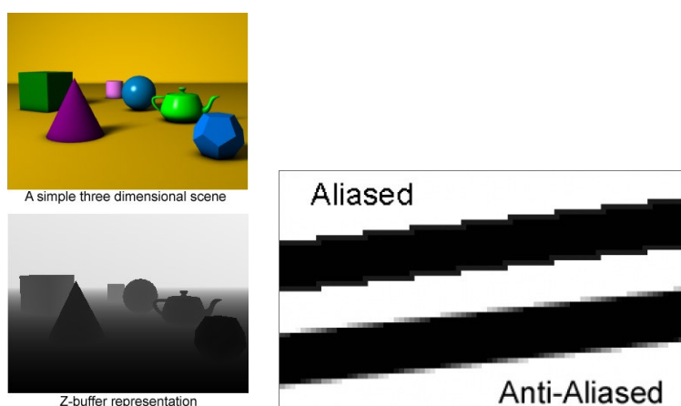
À gauche : une scène 3D et son Z-buffer. À droite : un bord crénelé (« aliased ») et anticrénelé.
